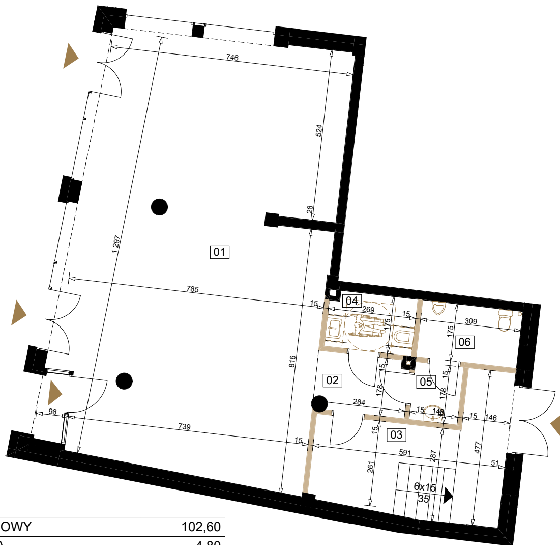
rzut kondygnacji
